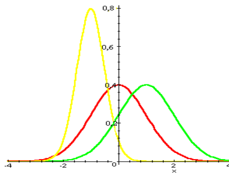
II.4.6. ábra Az N(-1, 0,5) , N(0, 1) és N(1, 1) normális eloszlások sűrűségfüggvényei
