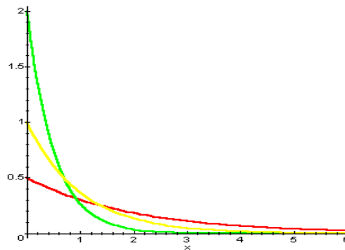
II.4.4. ábra A \lambda = 1, 2, 0,5 paraméterű exponenciális eloszlások sűrűségfüggvényei
