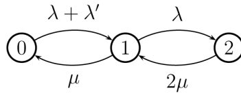
9.2. ábra. Melegtartalék
