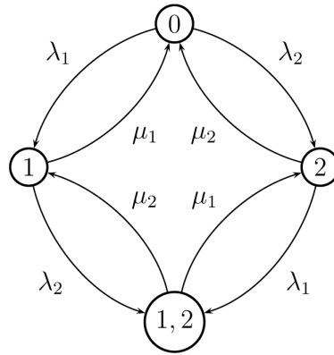
4.4. ábra. A 41. példa állapot átmenet diagramja
